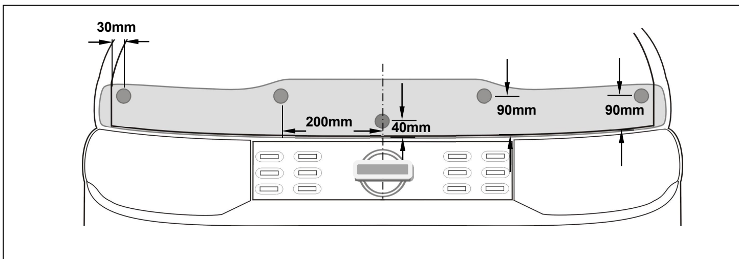
Illustration n°1 - Emplacements des butées
