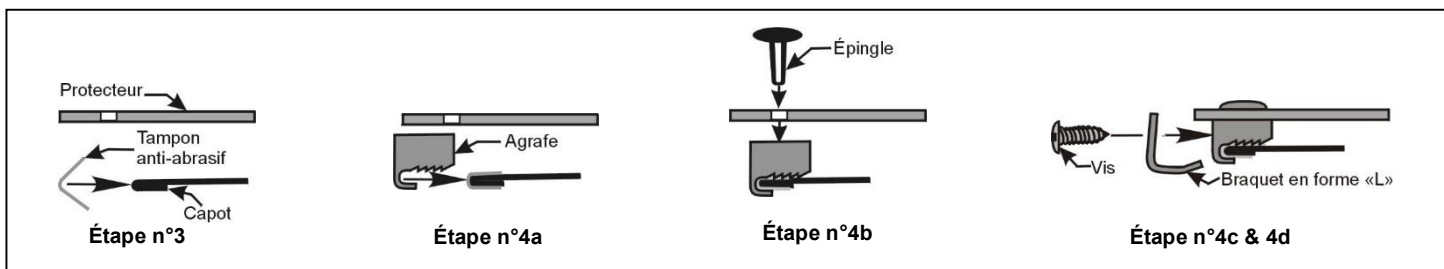
Illustration n°2 - Configuration de l'agrafe – N° de brevet : 6,892,427
